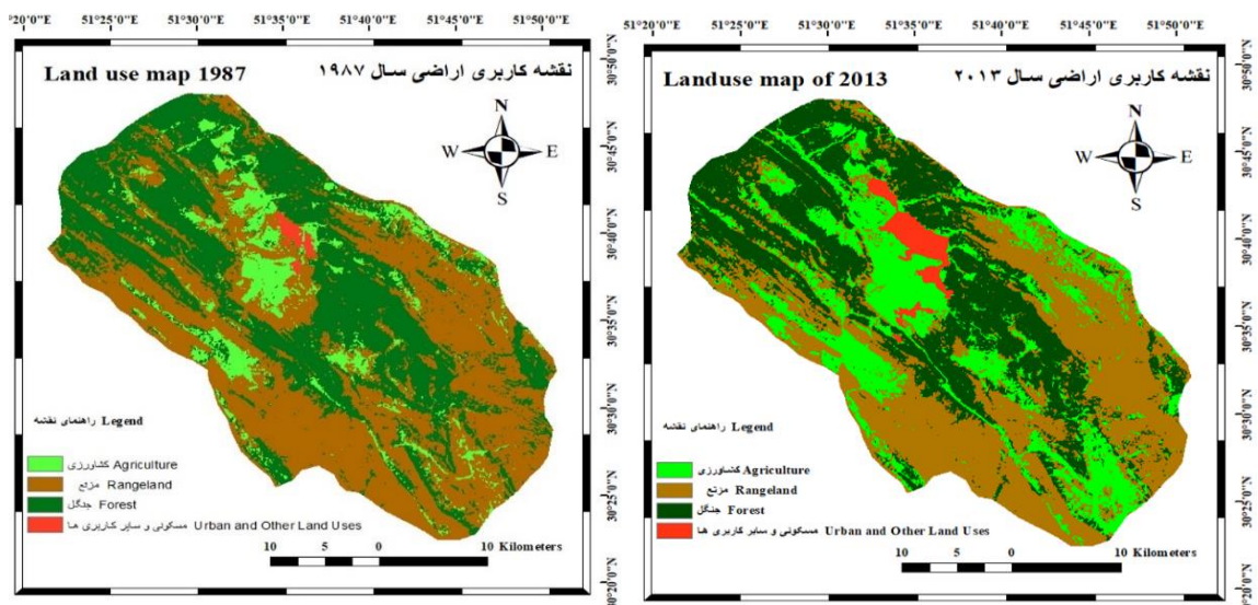
شکل ۲- نقشه کاربری اراضی منطقه مورد بررسی در سال‌های ۱۳۶۶ و ۱۳۹۲
