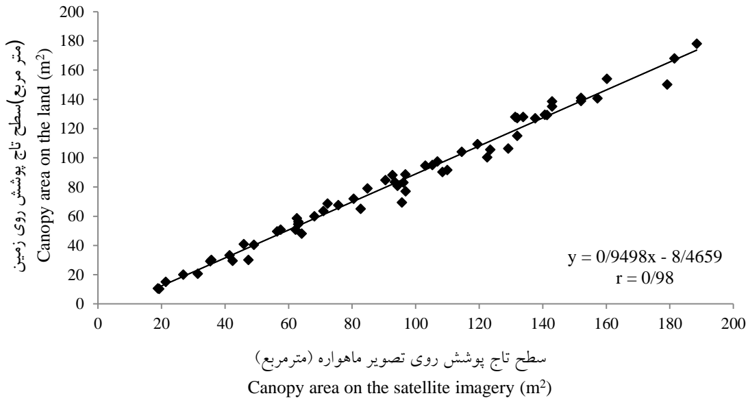
شکل ۳- رابطه خطی حاصل از مساحت اندازه‌گیری زمینی و تصاویر ماهواره در خیابان جمهوری اسلامی
