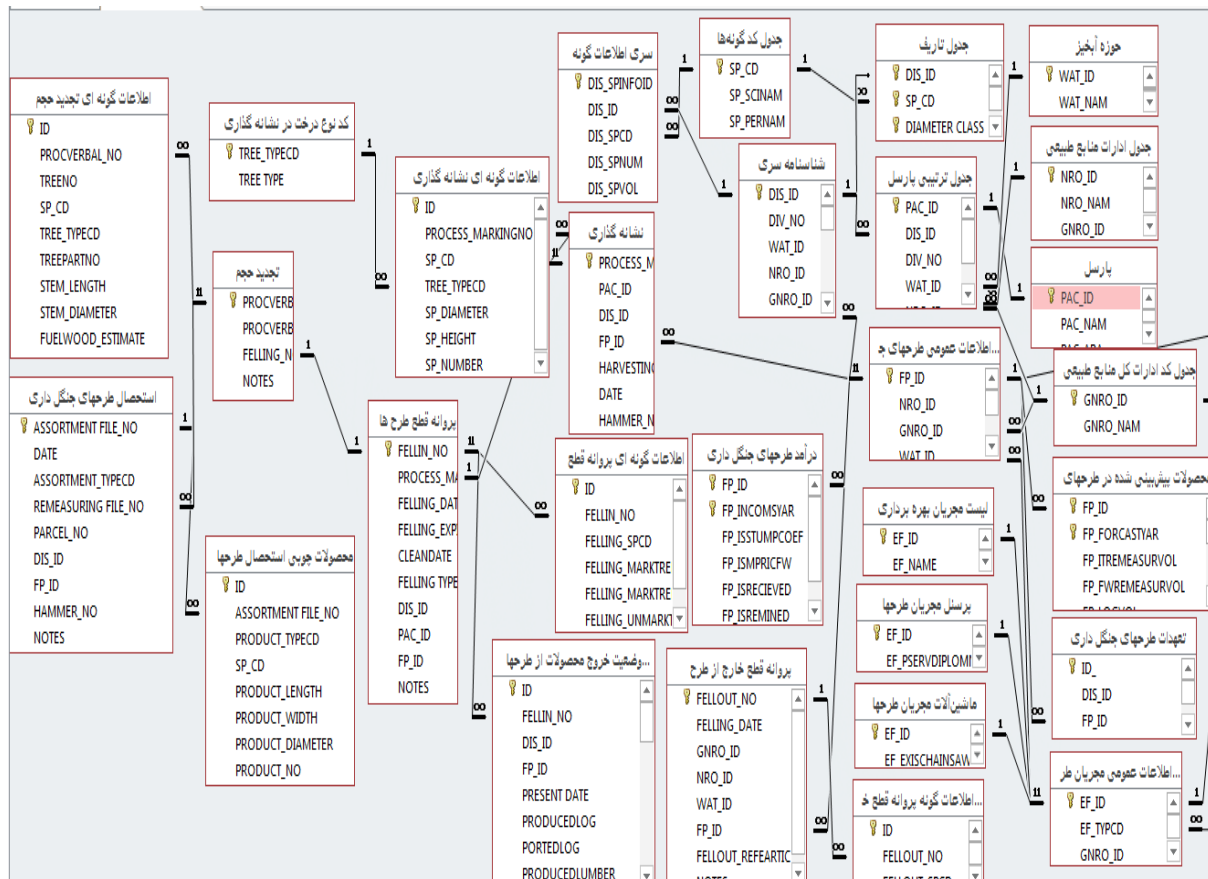
شکل ۲- دیاگرام موجودیت - رابطه، انواع روابط یا جداول و ویژگی‌های آن‌ها برگرفته از نرم‌افزار اکسس ۲۰۱۶
