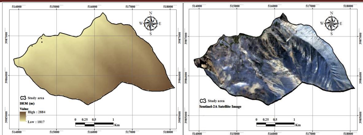
شکل ۴- مدل رقومی ارتفاع (سمت راست) و تصویر ماهواره‌ای سنتینل ۲ منطقه مورد بررسی (سمت چپ)
